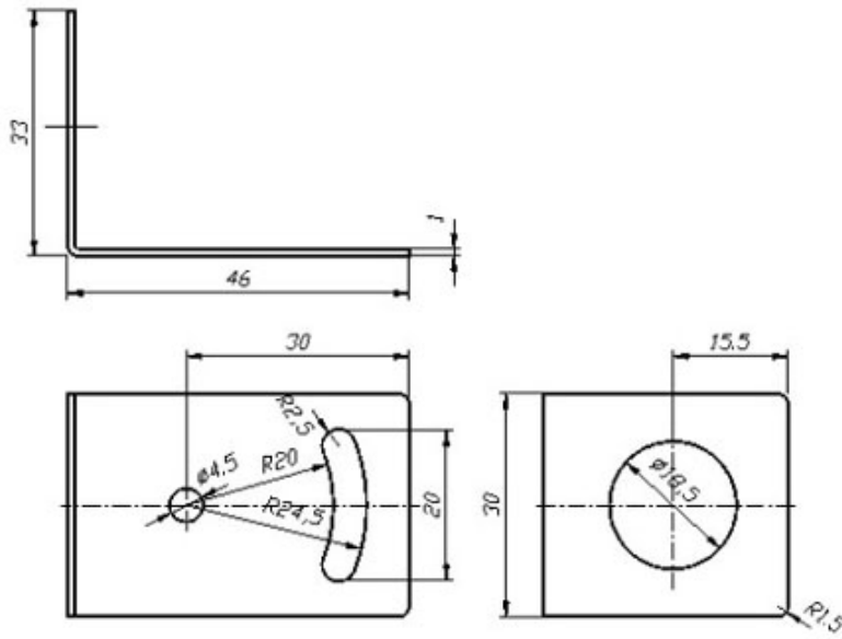
Кронштейн М 18.2
